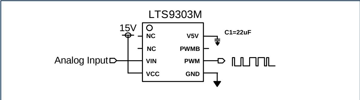
LTS9303 电压转PWM关系
