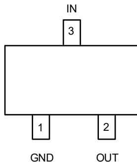
SOT23-3
