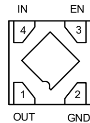
DFN1×1-4/UTDFN1×1-4
