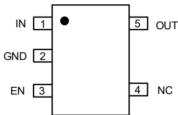
SOT23-5/SC70-5
